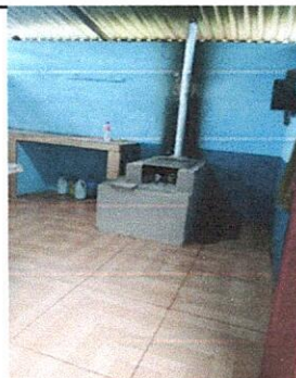
Foto 5: Sustrucción de estufa rural con chimenea, plancha y accesorios.
