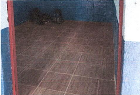
Foto1: Sustrucción de piso, por piso cerámico en áreas de aulas, dirección, bodega y corredor.
